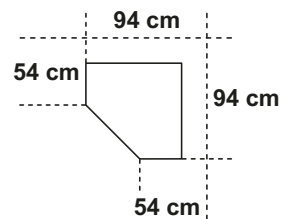
Stellskizzen für Eckschränke Art. 650
